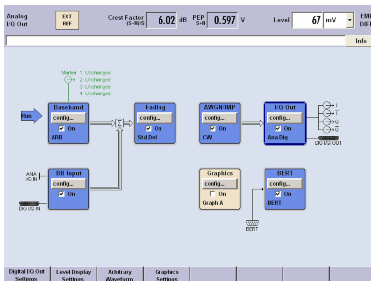
図 3-4: ベースバンド・メイン・モジュール 1 台とベースバンド・ソース 2 台を搭載した R&S AMU
