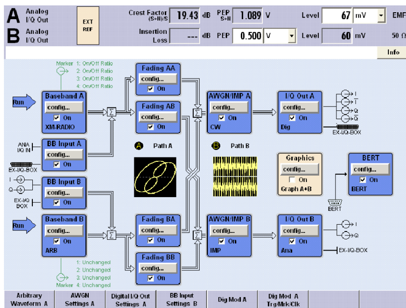
図 3-5: 2 パスとすべての機能を搭載した R&S AMU
