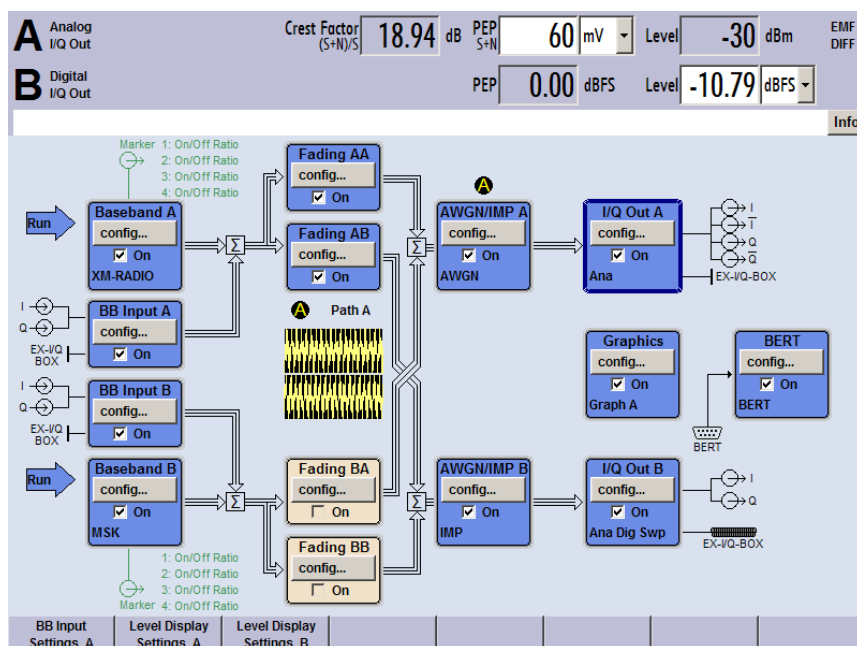
図 3-1: すべての機能を装備した R&S AMU のブロック・ダイアグラム
