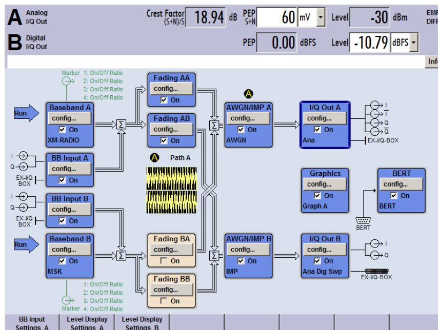
図 4-1: すべての機能を装備した R&S AMU のディスプレイ
